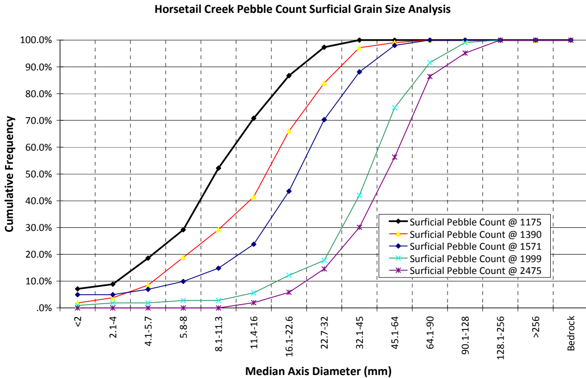
Figure 21. Surficial pebble count data.
